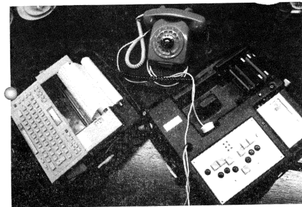
Dialogos-laitteisto koostuu kolmesta osasta: nauhurista (kuvassa oikealla), pistepuhelimesta (kuvassa samassa laatikossa nauhurin kanssa) sekä kirjoituskoneesta (kuvassa oikealla). Tavallisen puhelimen avulla Dialogos voidaan kytkeä toiseen samanlaiseen laitteeseen missä tahansa puhelinyhteyden päässä.
